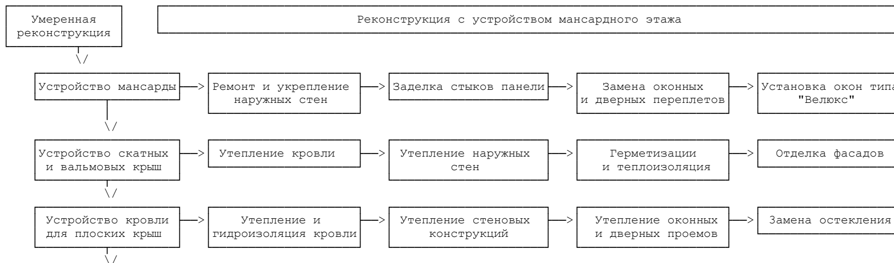
Рис. 2.1. Пример реконструкции жилого здания первого поколения с надстройкой мансар этажей без расселения (жирным шрифтом выделены работы по капитальному ремонту)
